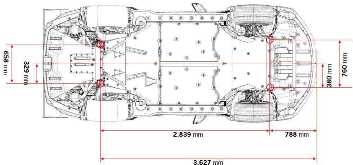
Positionen Fahrhöhenmesspunkte/ ride height measuring positions
